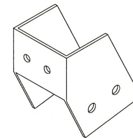
AXONOMETRIA UNIÓ TIPUS 10. XAPA PLEGADA D' ACER A42 e= 5mm
