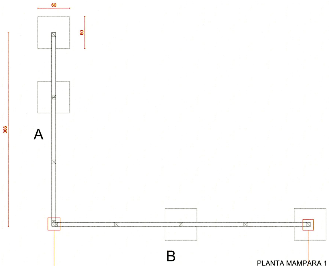
PLANTA MAMPARA 1
