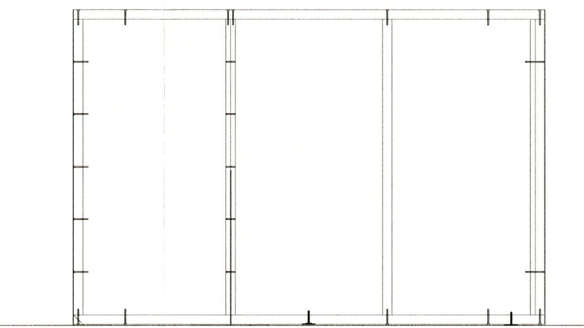
ALZADO A (BASTIDOR)
